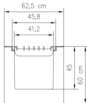
Stopprinne SR 400 G
